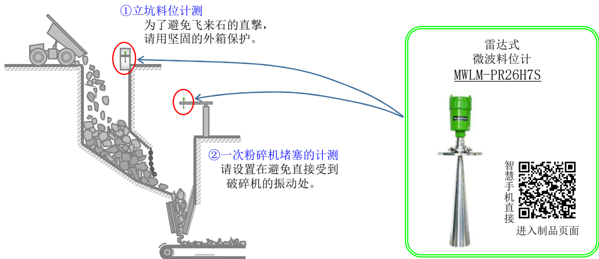
※图：矿山的立坑、一次粉碎机的料位，使用微波料位计的计测示意图。
